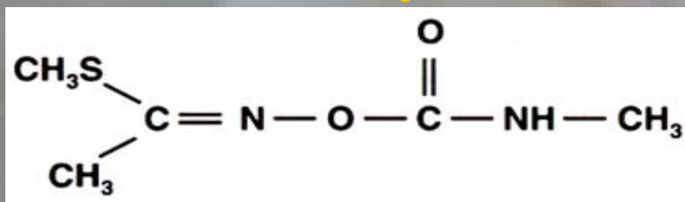
Methomyl
