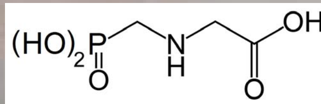
Glyphosate
