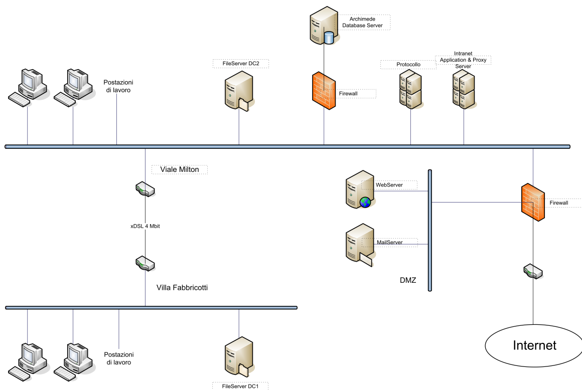
Figura 1: Descrizione dell'infrastruttura
